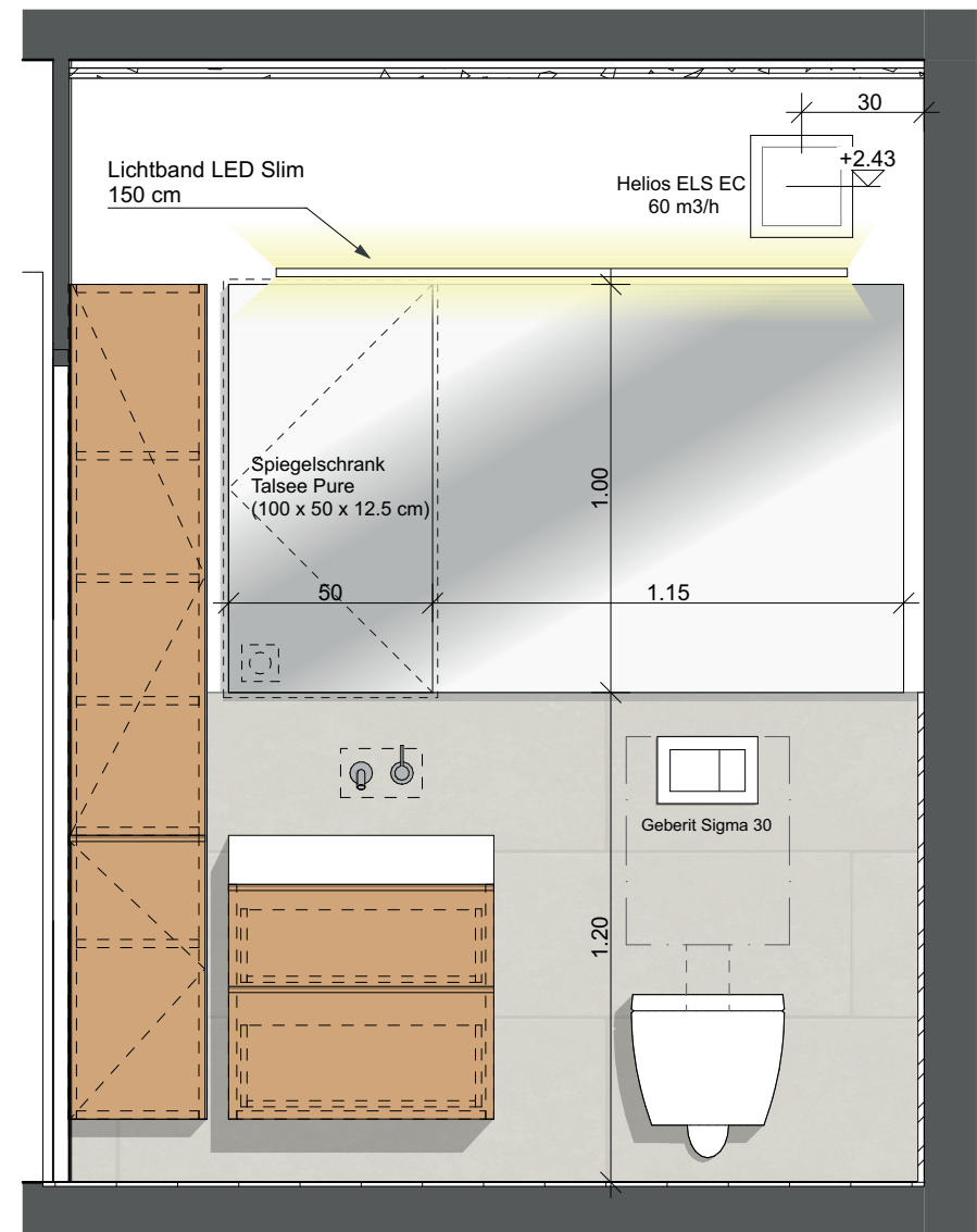
Ansicht
