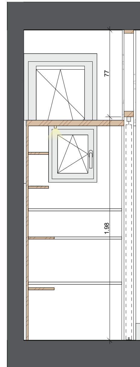
Schnitt E-E
