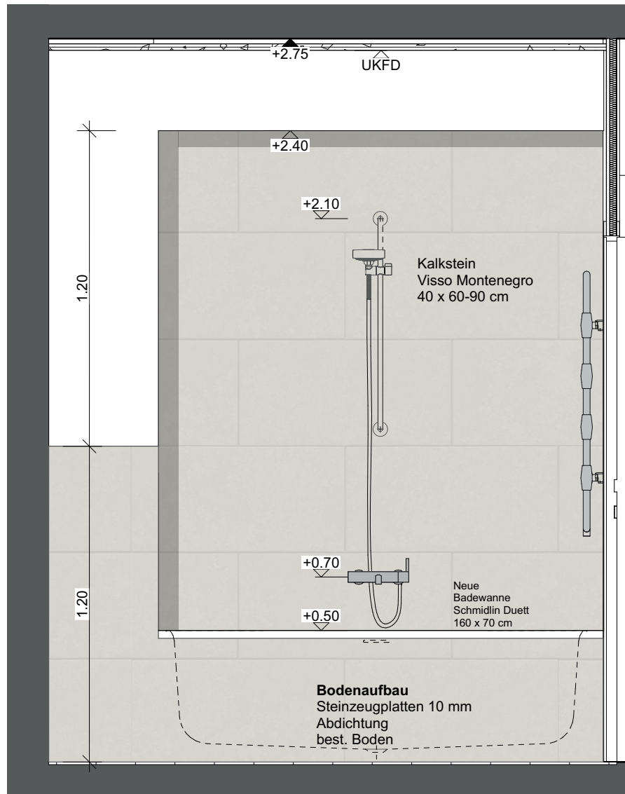
Ansicht
